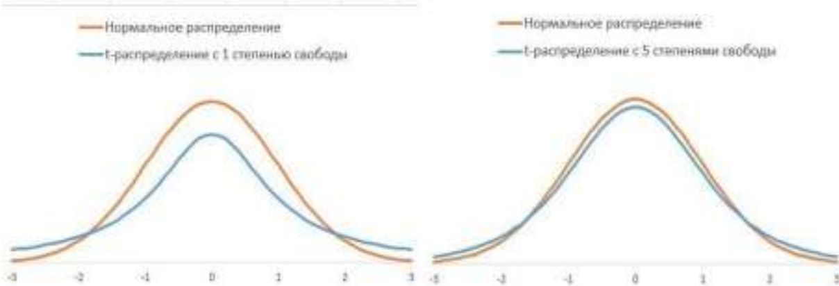
Рис. 2.4. Стандартизованное нормальное распределение и t -распределение Стьюдента с различным числом степеней свободы
