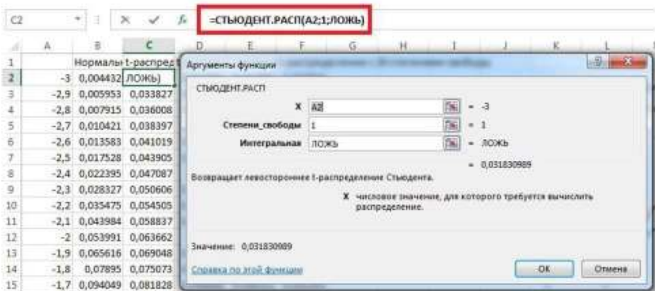
Рис. 2.5. Функция Excel =СТЮДЕНТ.РАСП() для построения плотности вероятности
