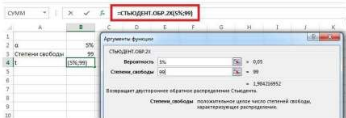
Рис. 2.8. Использование функции =СТЮДЕНТ.ОБР.2Х() для определения t -параметра по известной вероятности (обратная задача построению плотности распределения)
