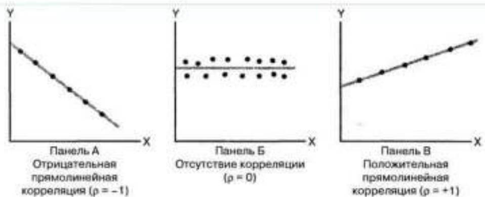
Рис. 6.2. Примеры зависимости между двумя переменными
