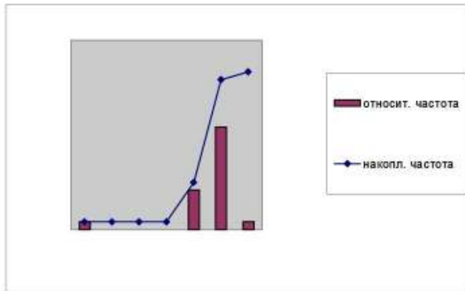
Рисунок 3.9. Гистограмма и кумюлята относительных частот
