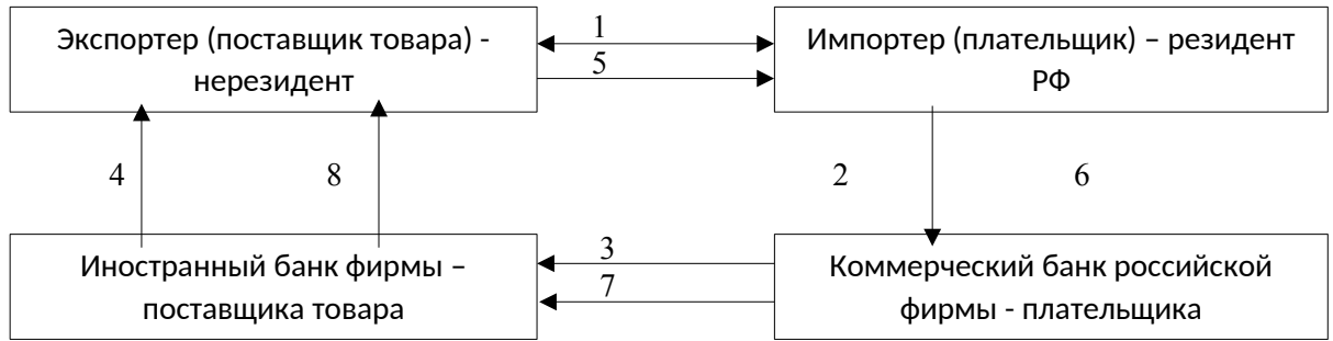
Рис. 1.Схема документооборота
