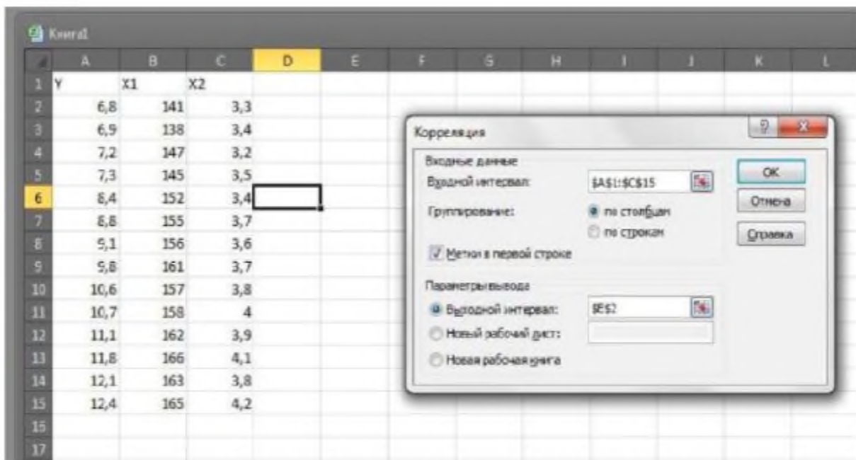
Рис. 7.1. Заполнение окна «Корреляция»
