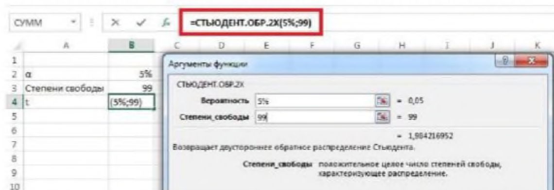
Рис. 2.8. Использование функции =СТЮДЕНТ.ОБР.2Х() для определения t -параметра по известной вероятности (обратная задача построению плотности распределения)
